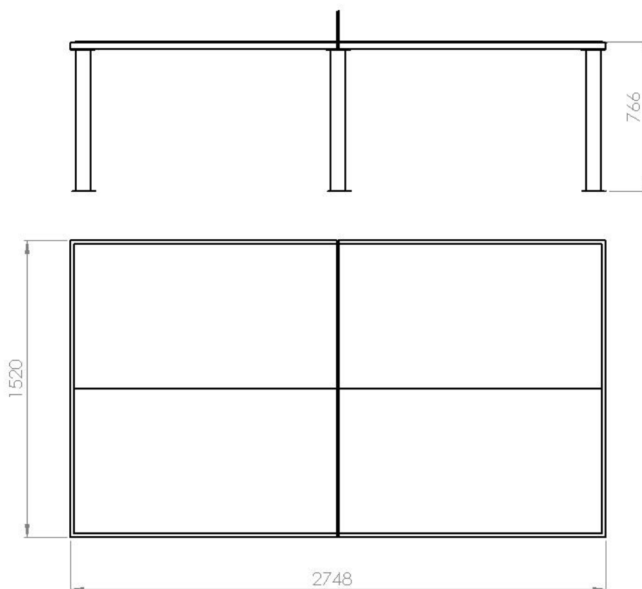
ТЕНИС МАСА РАЗМЕРИ В ММ
